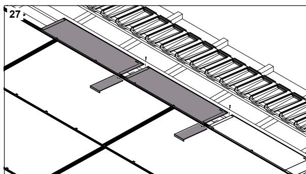
Stossbleche einschieben und mit Breitkopfstift fixieren, weitere Firstbleche verketten
