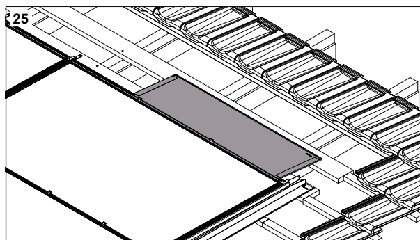
Firstblech einlegen
