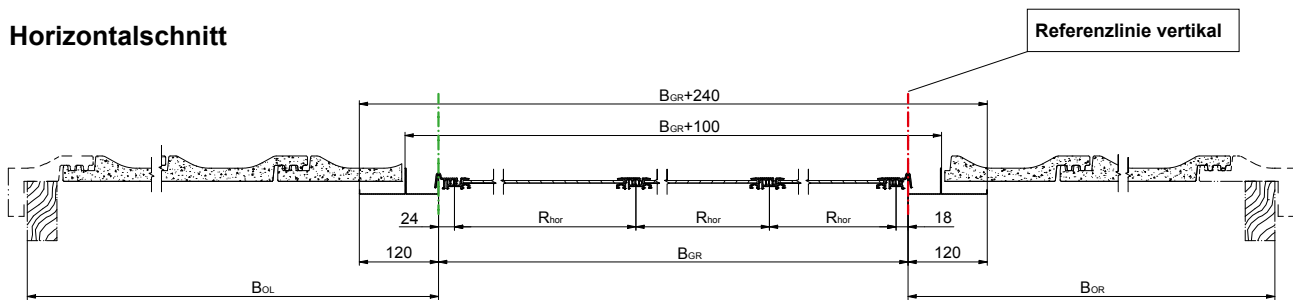
Abbildung: Horizontalschnitt Solrif
