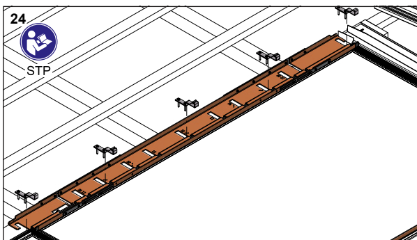
Oberste Profilbügelreihe verlegen
